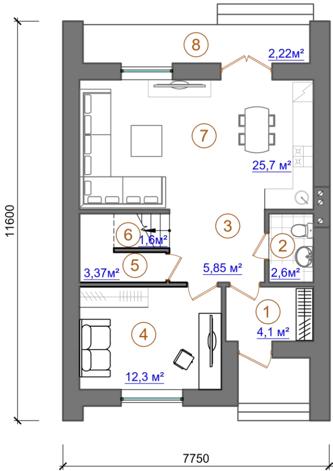
План 1-го поверху
