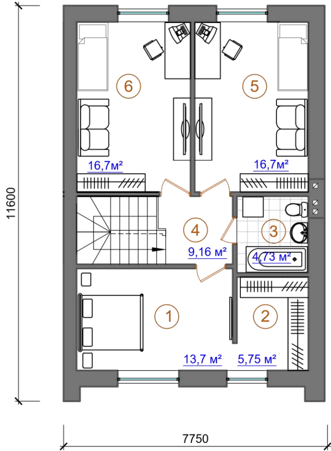
План мансардного поверху
